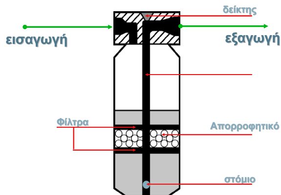
Τομή ξηραντήρα
